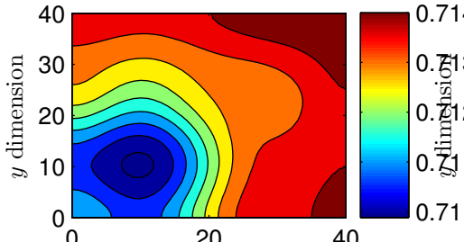
u(x, 10).
