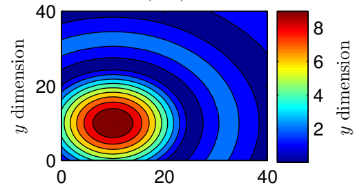
u(x, 0).
