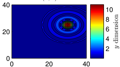
v(x, 0).
