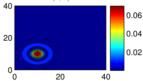
r(x, 0).
