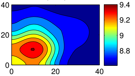
r(x, 10).
