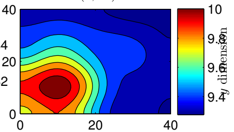
w(x, 10).
