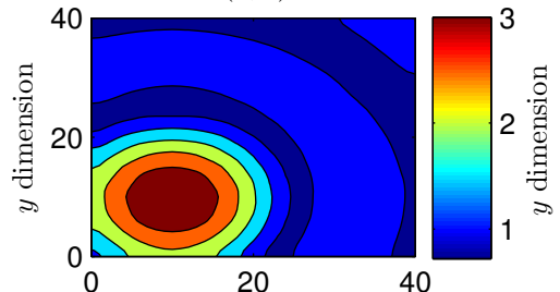
u(x, 1).
