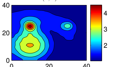
r(x, 1).
