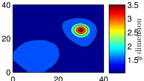
v(x, 1).
