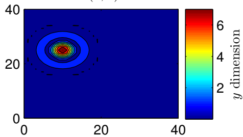
w(x, 0).
